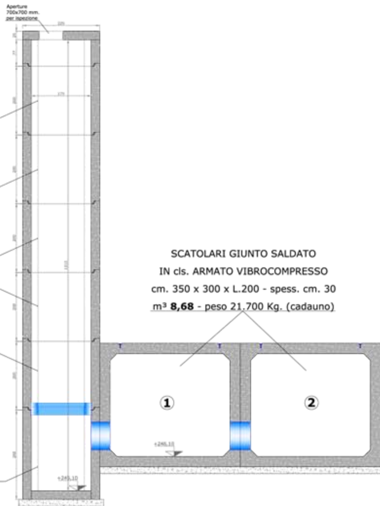
SEZIONE D-D 1:50
