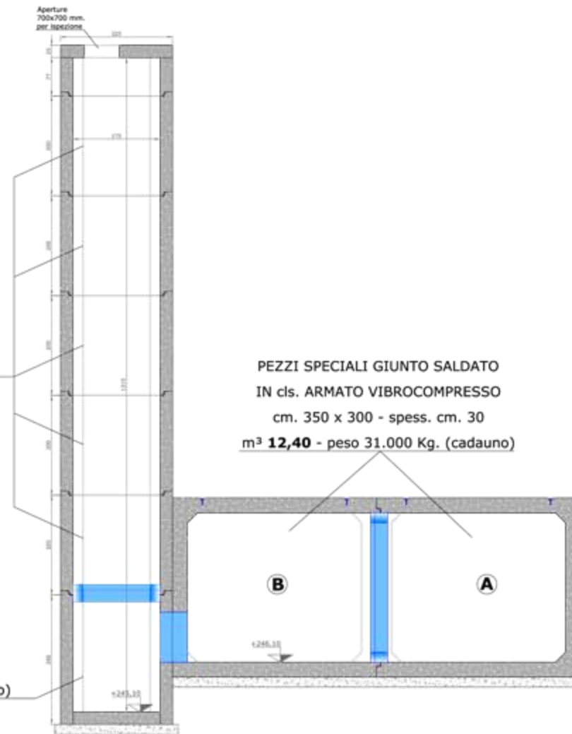
SEZIONE C-C 1:50
